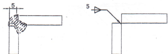
Double - Fillet
